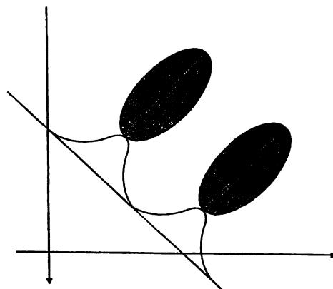
Figura 13.3. Representación de la dirección óptima de proyección para discriminar entre las dos poblaciones.
