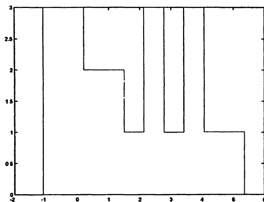
Figura 11.2. Histograma de la segunda variable en la mezcla de normales.
