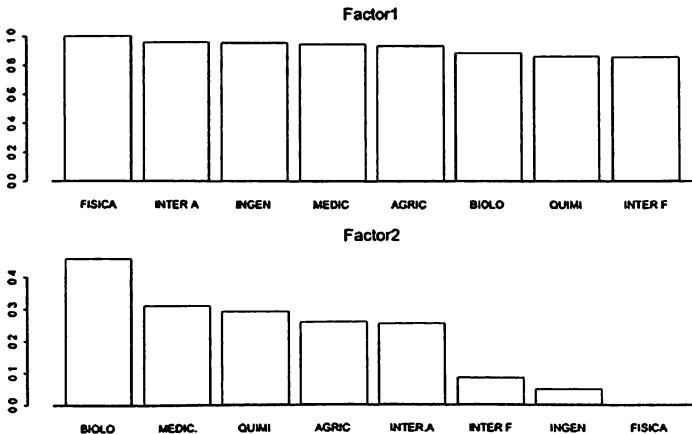
Figura 12.2. Pesos de los variables de INVEST en los dos factores estimados por MV.
