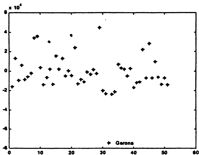
Figura 4.20. Tercera proyección en la dirección de máxima kurtosis para los datos de la EPF.
