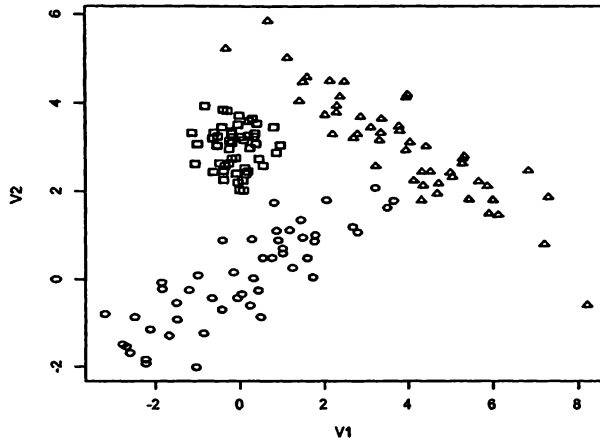
Figura 15.7. Solución final para los datos de Diday.
