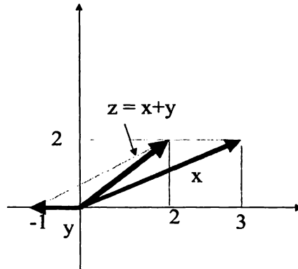
Figura 2.1. Suma de dos vectores.
