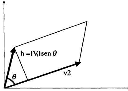
Figura 2.4. El valor absoluto del determinante como área del paralelogramo formado por los dos vectores.
