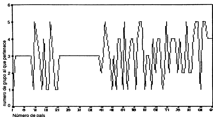
Figura 8.9. Indicación de los países que pertenecen a cada uno de los grupos.
