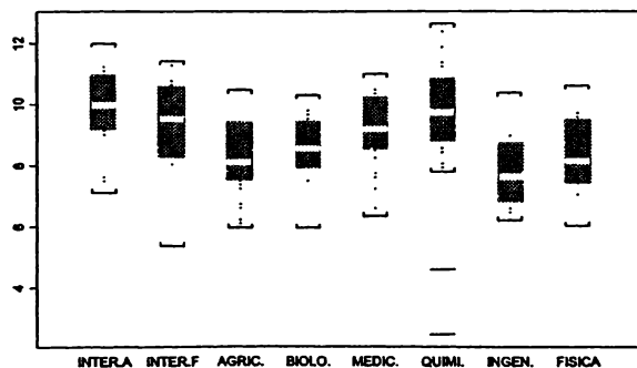
Figura 5.8. Diagrama de cajas de los logaritmos de las variables de INVEST una vez eliminado Estados Unidos.
