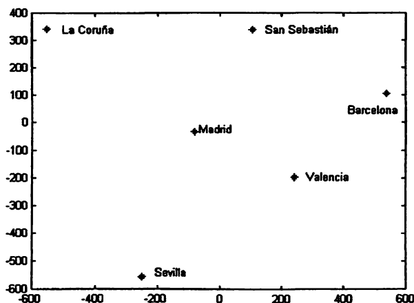
Figura 6.1. Representación de las coordenadas principales de seis ciudades españolas.
