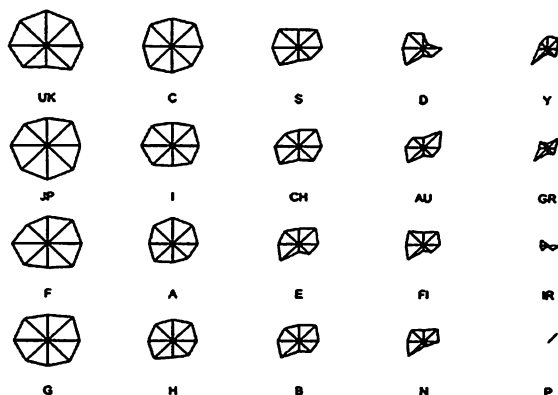
Figura 4.10. Representación mediante estrellas de los países de INVEST en logaritmos una vez eliminado Estados Unidos.
