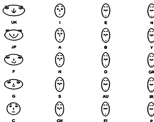
Figura 4.8. Representación de las contribuciones científicas de los países de INVEST en caras de Chernoff.
