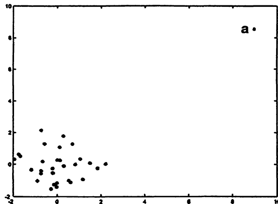
Figura 4.15. Las variables estaban originalmente casi incorreladas ( r = -.11 ), pero la presencia del valor atípico, \mathbf{a} , ha creado una fuerte correlación positiva ( r = .71 ).
