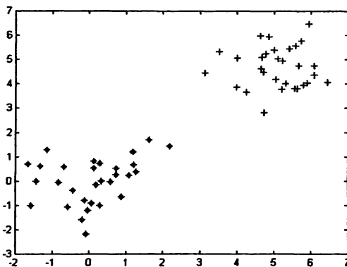
Figura 8.12. Dos grupos con variables incorreladas dentro de los grupos pueden dar lugar a una alta correlación aparente entre las variables.
