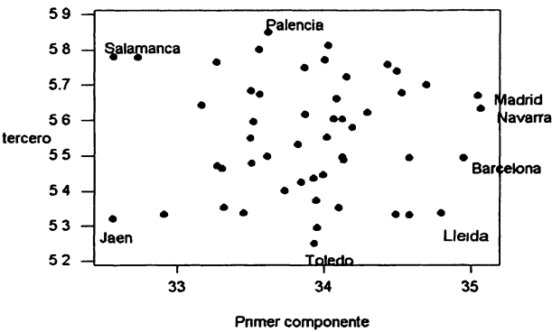
Figura 5.3. Representación de los datos de la EPF en el plano definido por los componentes primero y tercero.
