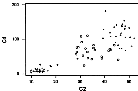
Figura 8.11. Resultados de k-medias para datos estandarizados de MUNDODES con el programa Minitab. En ordenadas la mortalidad infantil (C4) y en abscisas la tasa de natalidad (C2).
