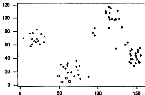
Figura 8.4. División de los datos de Ruspini en cuatro con Minitab.
