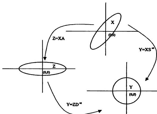
Figura 5.4. Representación gráfica de la relación entre componentes principales y estandarización multivariante.
