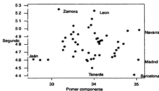
Figura 5.2. Proyección de los datos de la EPF sobre el plano definido por las dos primeras componentes principales.
