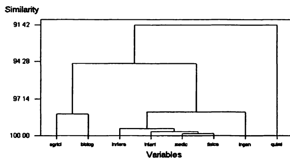
Figura 8.20. Dendrograma para las variables de INVES con el criterio de Ward.
