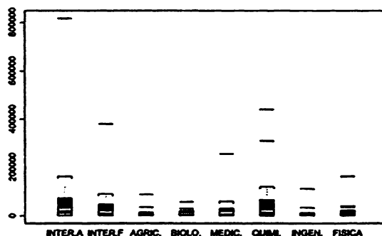
Figura 4.11. Diagrama de cajas de las variables de INVEST.
