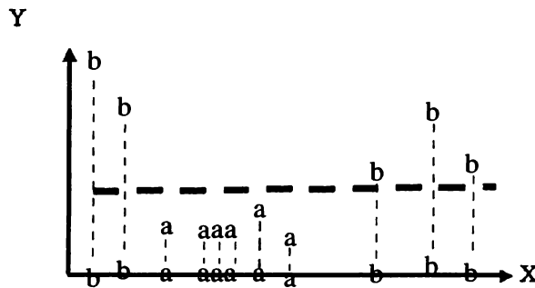
Figura 14.5. Los puntos a y b no son linealmente separables en la dimensión X pero sí lo son en el plano.
