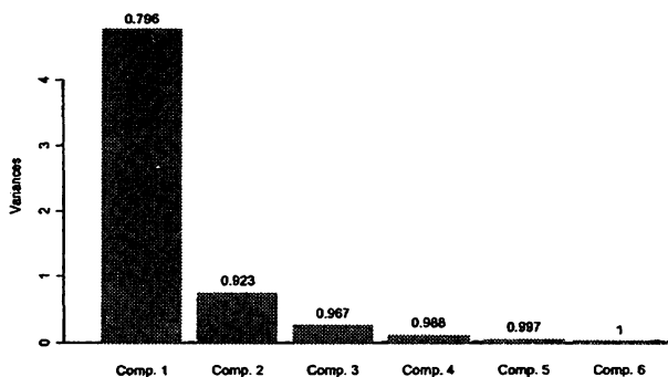
Figura 5.14. Proporción de variabilidad explicada por cada componente para los datos de MUNDODES.
