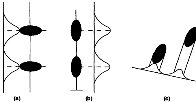
Figura 13.4. En los casos (a) y (b) la dirección óptima coincide con la línea de medias y con los ejes de la elipse. En el caso (c) es un compromiso entre ambos.
