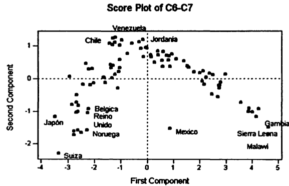
Figura 5.16. Representación de los dos primeros componentes para los datos de MUNDODES.
