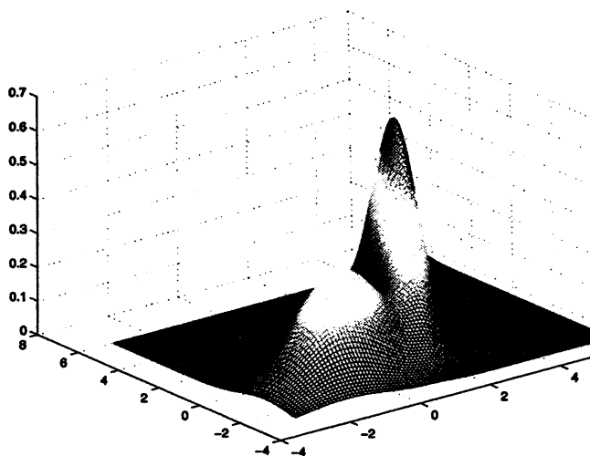
Figura 9.9. Mezcla de dos normales bivariantes en la proporción 50 por 100 con medias (0,0) y (3,3) y distintas matrices de covarianzas.
