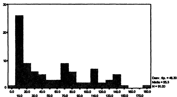
Figura 15.1. Histograma de la variable mortalidad infantil indicando la presencia de entre cuatro y cinco grupos de países.
