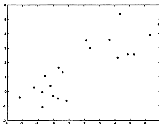
Figura 11.3. Diagrama de dispersión de las dos variables.
