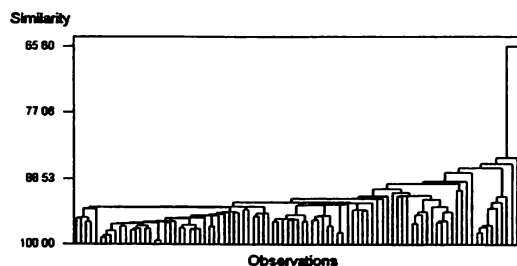
Figura 8.16. Resultados de una aglomeración jerárquica para los países de MUNDODES con encadenamiento simple.
