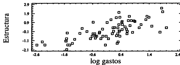
Figura 16.2. Relación de la estructura del hogar con el logaritmo de los gastos.
