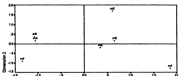
Figura 6.5. Representación de los productos con el escalado no métrico.
