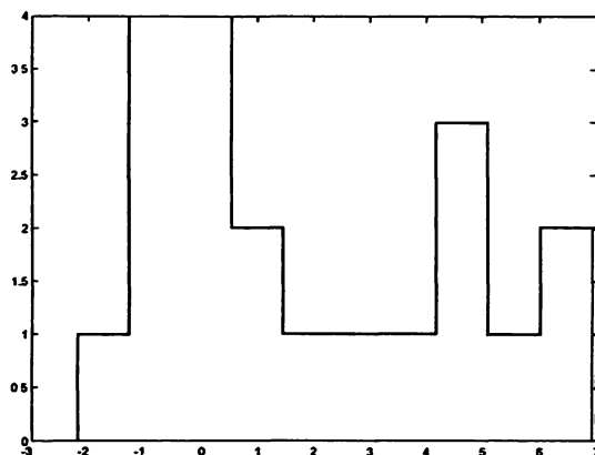
Figura 11.1. Histograma de la primera variable de la mezcla de normales.
