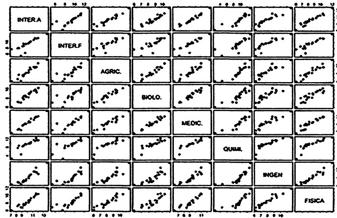
Figura 4.6. Matriz de gráficos de dispersión para los datos de INVES.
